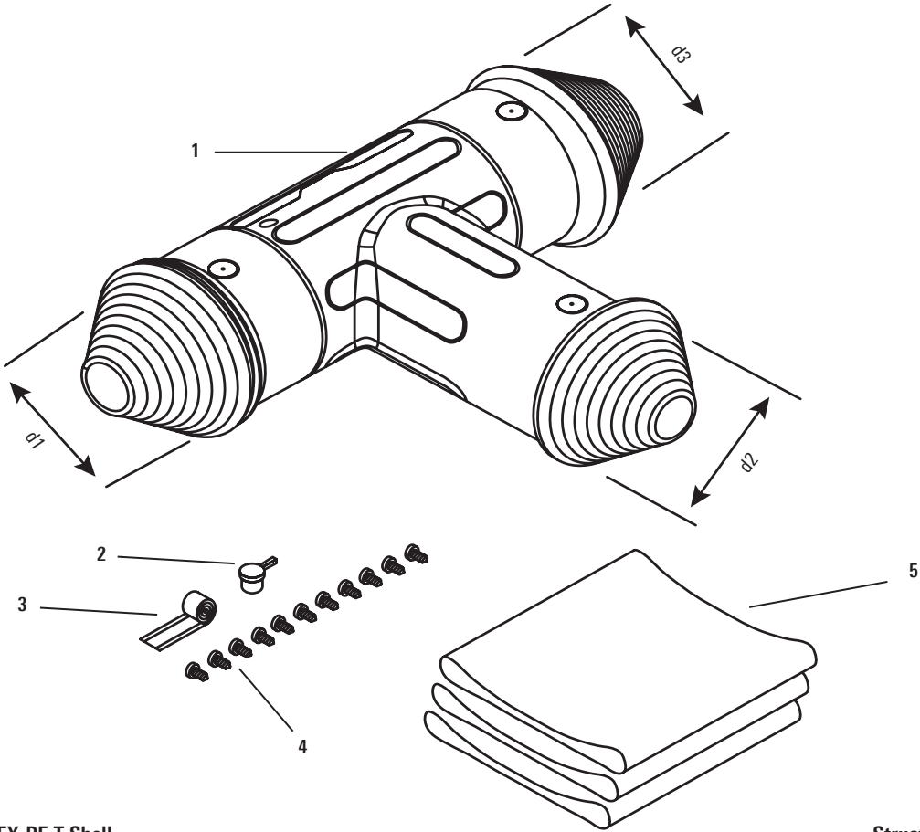
CALPEX-PE-T-Shell
