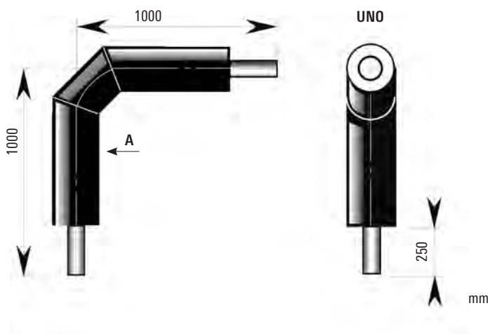
Dimensions Ø 125 - 315 mm / SDR 11
